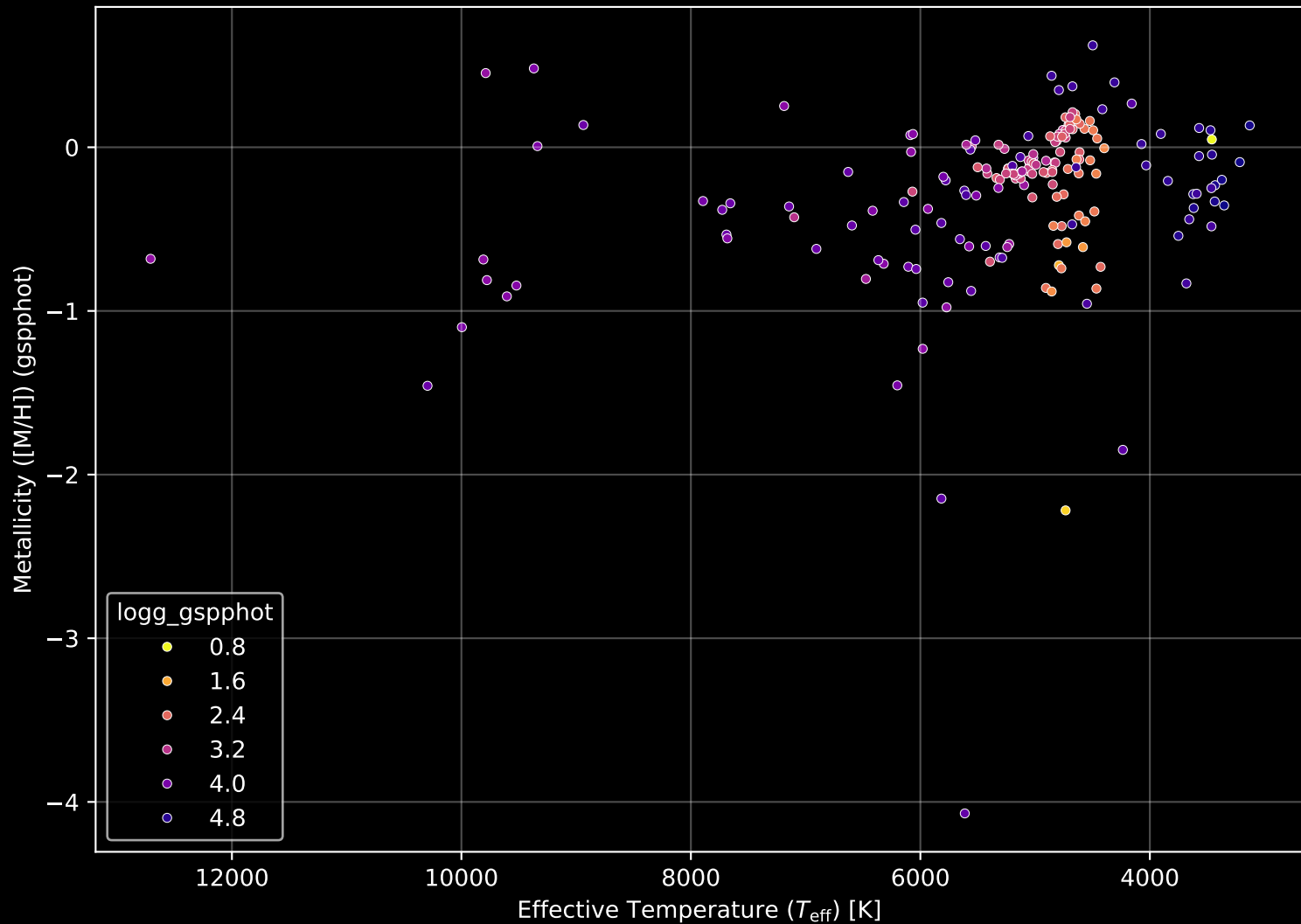
APOGEE DR17 Field: [K2_C7_016-13_btx] Stellar Population Parameters (n= 189)
